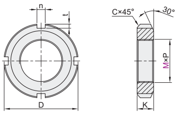
圆螺母 TBK74 TBK75
