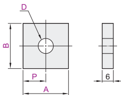
单孔型 TBL51/52/56
