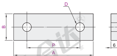
双孔型 TBL71/72/76
