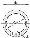
挡圈尺寸
