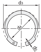
挡圈尺寸
