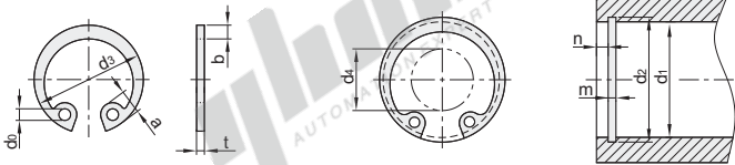
挡圈尺寸
