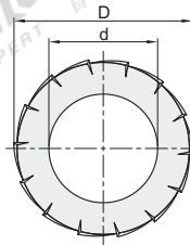
外锯齿型垫圈 TBY35
