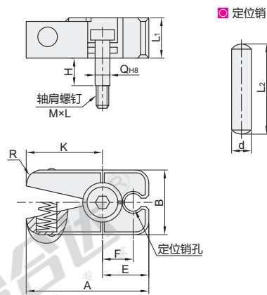
紧凑型 TFC72
