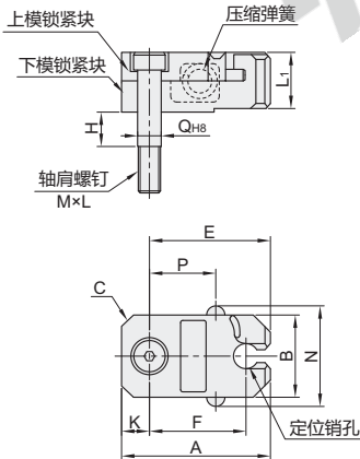
标准型 TFC71
