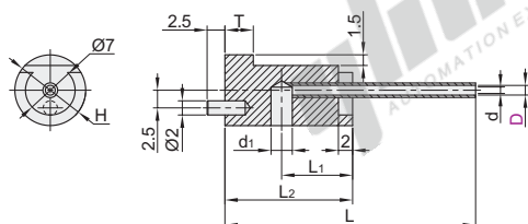
肩定位型 TFD43
