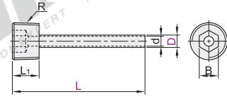
锥螺纹型 TFD45
