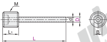
直螺纹型 TFD44
