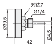
螺钉型 TFD55
