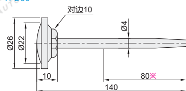
探针型 TFD56
