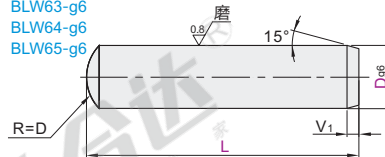
标准型·公差h7/g6
