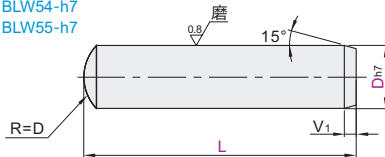
标准型·公差h7
