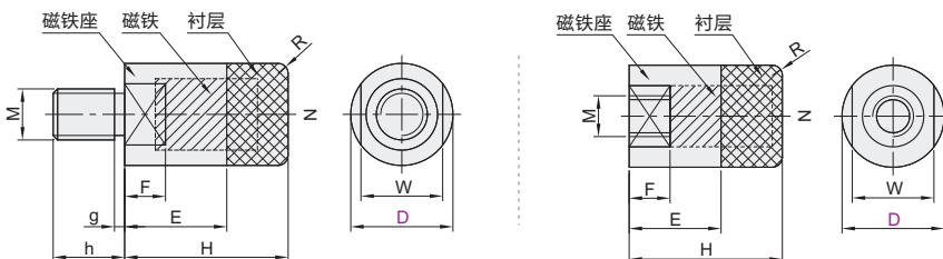
外螺纹型 BMQ51/56
