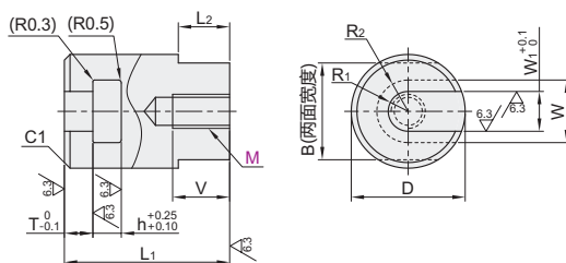
嵌入型·内螺纹型 WHN11/12
