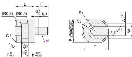
嵌入型·外螺纹型 WHN01/02
