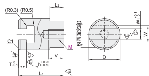
通孔型·内螺纹型 WHN41
