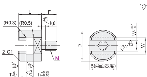
通孔型·外螺纹型 WHN31/32
