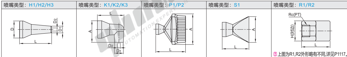
② 喷嘴选择(表2)
