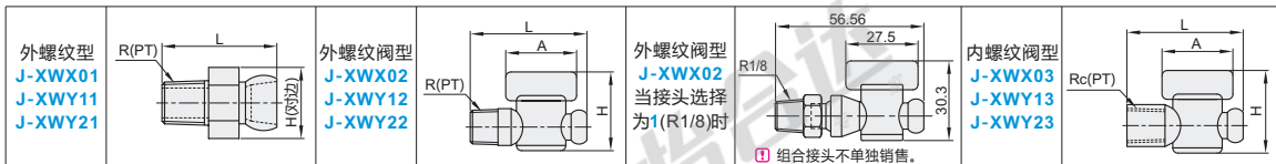
① 接头选择(表1)
