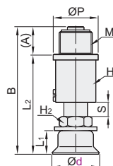
弹簧式直接安装型 J-WES81/82
