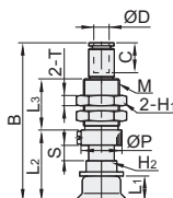
弹簧式顶部真空端口 J-WES66/67
