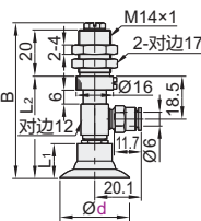
弹簧式侧面真空端口 J-WET71/72
