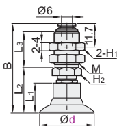
弹簧式侧面真空端口 J-WET71/72
