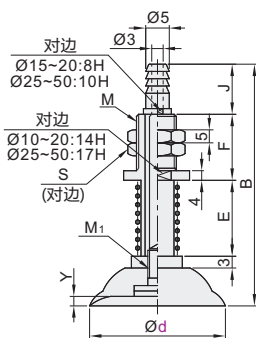
盘径Ø15-50
