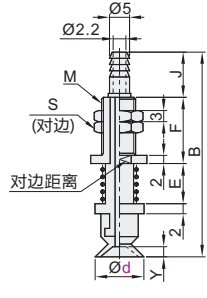
盘径Ø15-50
