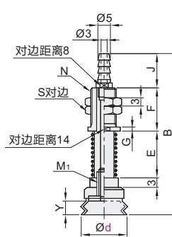
盘径 \phi 10\sim 50
