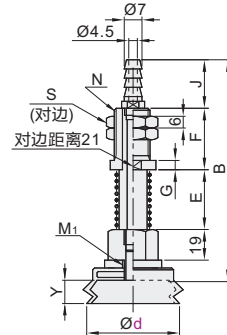
盘径 \phi 60\sim 80
