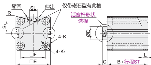
油路板型 WSA62
