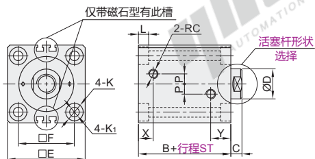
配管型 WSA61
