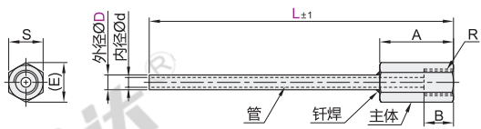
内螺纹 NHR02 公称型号：3/5/6
