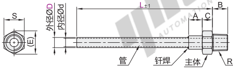
外螺纹 NHR01 公称型号：0.5/1
