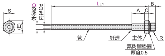
内螺纹 NHR02 公称型号：3/5/6
