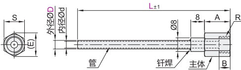
内螺纹 NHR02 公称型号：1
