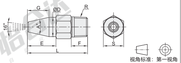
锥形 NHR66 NHR67
