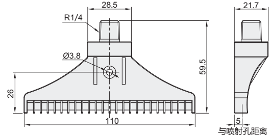
加宽型 NHR76
