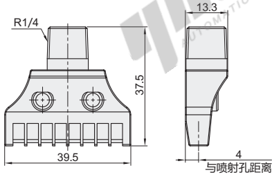
圆头型 NHR77
