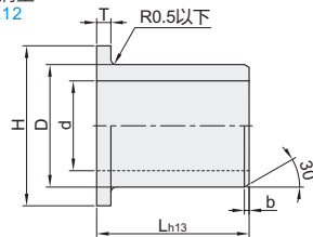
薄壁肩型 OBK12
