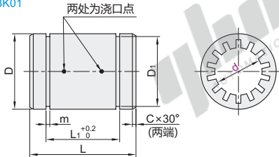
标准型 OBK01
