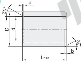
薄壁直柱型 OBK11
