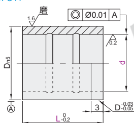
紧配型·直柱型 OFC41
