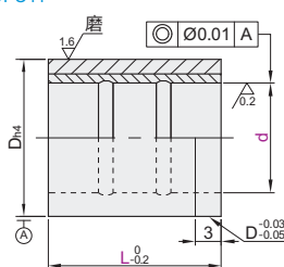
胶粘型·直柱型(材质: SUJ2+铜合金) OFC11
