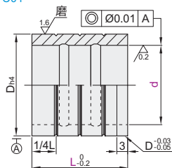
胶粘型·直柱型(材质: SUJ2) OFC01
