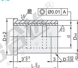
胶粘型·肩型(材质: SUJ2+铜合金) OFC12
