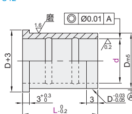
紧配型·肩型 OFC42
