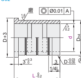
胶粘型·肩型(材质: SUJ2) OFC02
