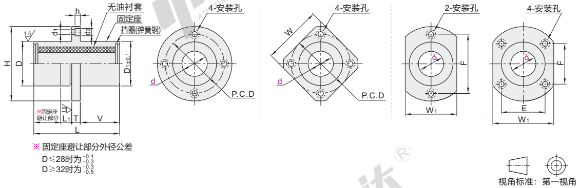
圆法兰型 OGJ01/02
