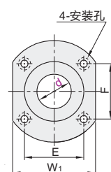
对边法兰型 OGJ61/62
