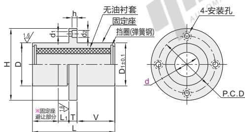
圆法兰型 OGJ01/02
