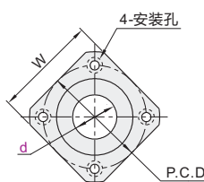
方法兰型 OGJ31/32
