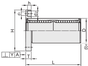
双衬型
