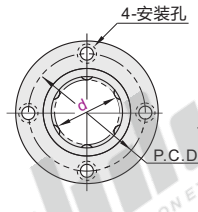
圆法兰型
