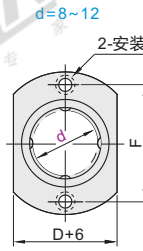
对边法兰型
