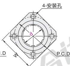
方法兰型 LML11/12
