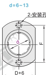
对边法兰型 LML21/22
