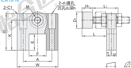
凹型限位块+聚氨酯螺钉 ICR15/16
