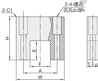
凹型限位块+定位螺栓 ICR11/12
