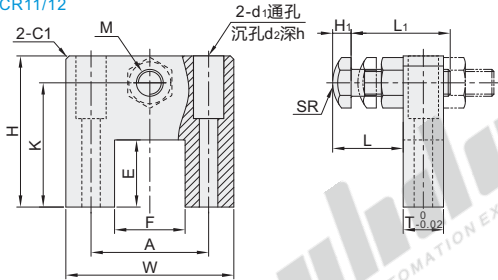
凹型限位块+定位螺栓 ICR11/12
