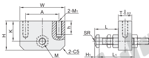
方型限位块+定位螺栓 ICR71/72
