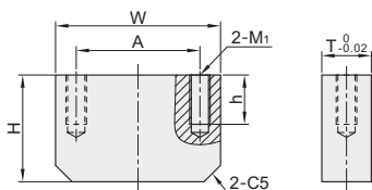
方型限位块(无孔) ICR61
