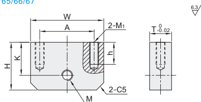
方型限位块(螺纹孔) ICR64/65/66/67
