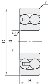
圆柱孔型
