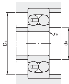
(安装图)
