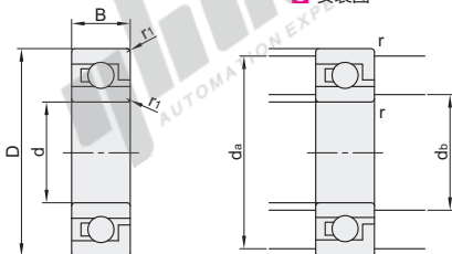
安装图
