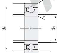
■ 安装图
