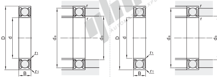
非接触式橡胶密封圈型
