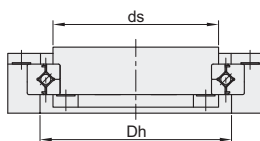
■ 安装图
