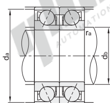
安装图
