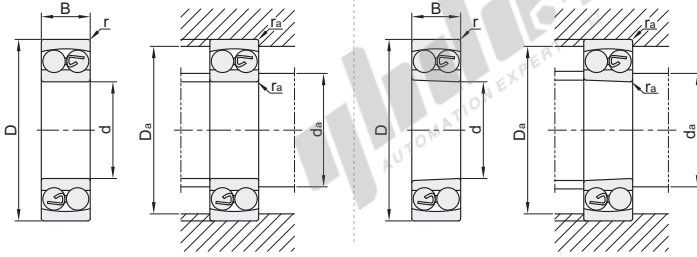
圆柱孔型
