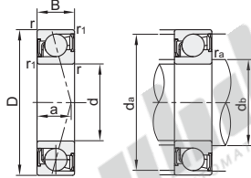
高速单列角接触球轴承 BBY06
