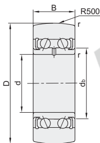
圆弧形 LR...-2RS
