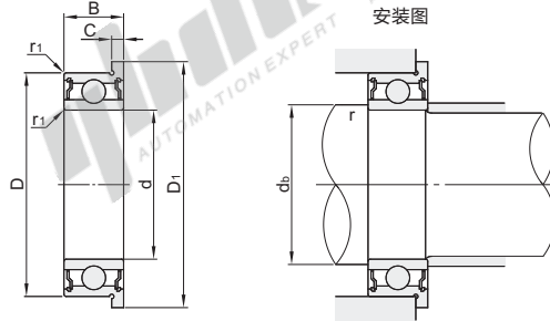
安装图
