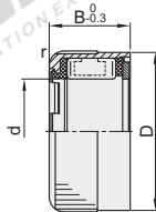
滑动轴承型(外形图B)
