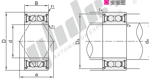
☑ 安装图
