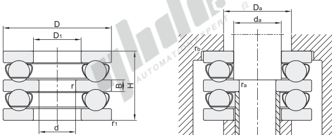
安装图
