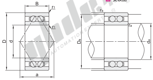
◎ 安装图
