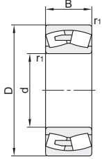
圆柱孔型
