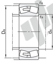
安装图
