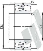
安装图
