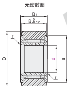
无密封圈
