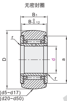
无密封圈
