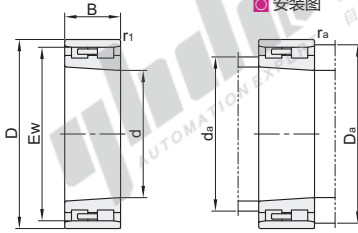
安装图
