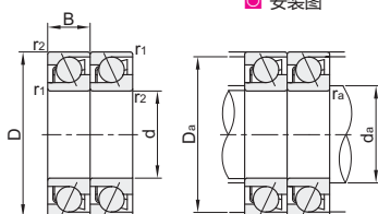
安装图
