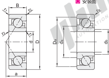
安装图
