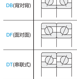
两个轴承组配安装图
